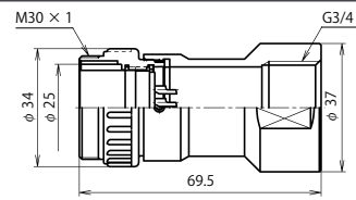
NJW-28 ■ -GAdF3/4 (注)
