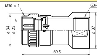
NJW-28 ■ -GAdM3/4 (注)
