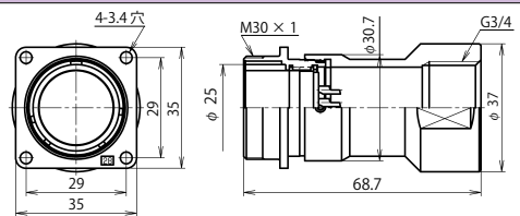
NJW-28 ■ -GAd(F)F3/4 (注)
