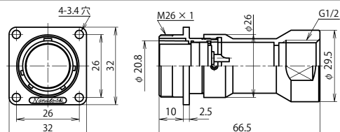
NJW-24 ■ -GAd(F)F1/2 (注)
