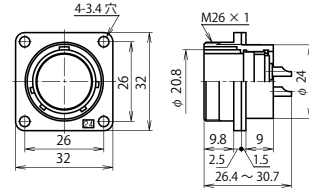
NJW-24 ■ -RF
