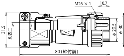
NJW-24 ■ -PMK □
