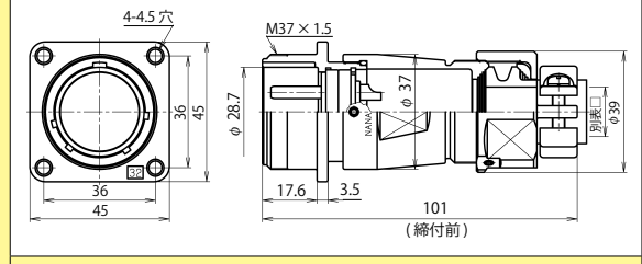
NJW-32 ■ -Ad(F)M □
