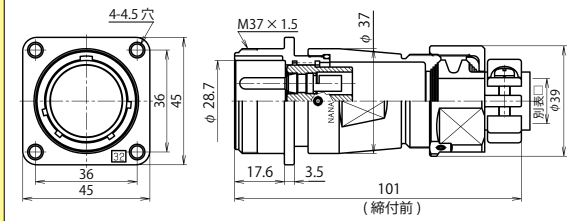
NJW-32 ■ -Ad(F)M □
