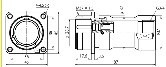
NJW-32 ■ -GAd(F)M3/4 (注)
