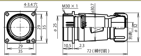
NJW-28 ■ -Ad(F)M □
