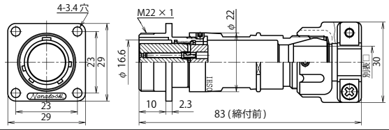
NJW-20 ■ -Ad(F)FK □
