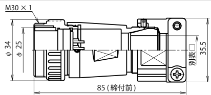
NJW-28 ■ -AdFK □
