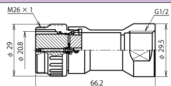
NJW-24 ■ -GAdF1/2 (注)
