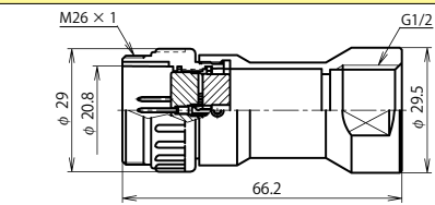
NJW-24 ■ -GAdM1/2 (注)
