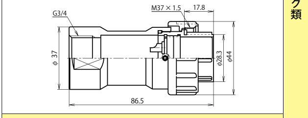
NJW-32 ■ -GPF3/4 (注)
