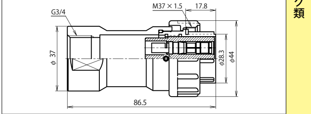
NJW-32 ■ -GPF3/4 (注)
