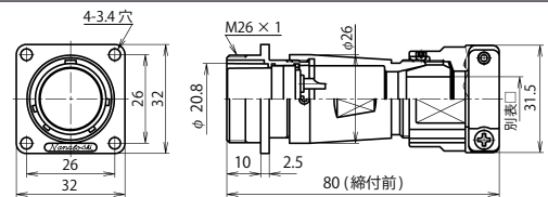
NJW-24 ■ -Ad(F)FK □
