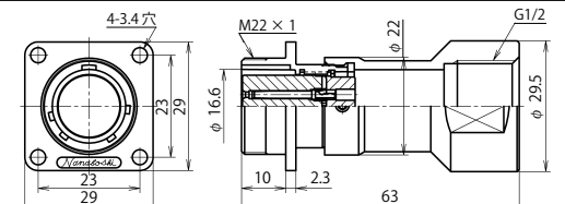
NJW-20 ■ -GAd(F)F1/2 (注)
