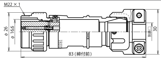
NJW-20 ■ -AdFK □
