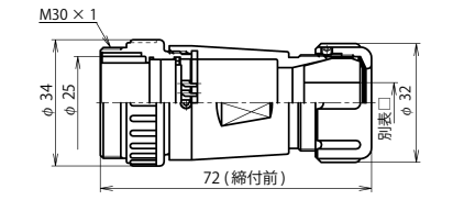
NJW-28 ■ -AdF □
