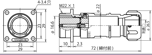
NJW-20 ■ -Ad(F) □
