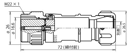
NJW-20 ■ -AdF □
