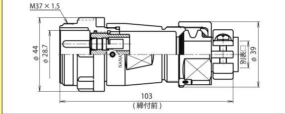
NJW-32 ■ -AdM □
