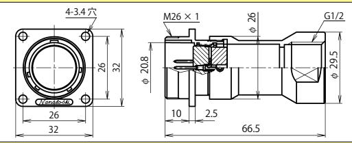
NJW-24 ■ -GAd(F)M1/2 (注)
